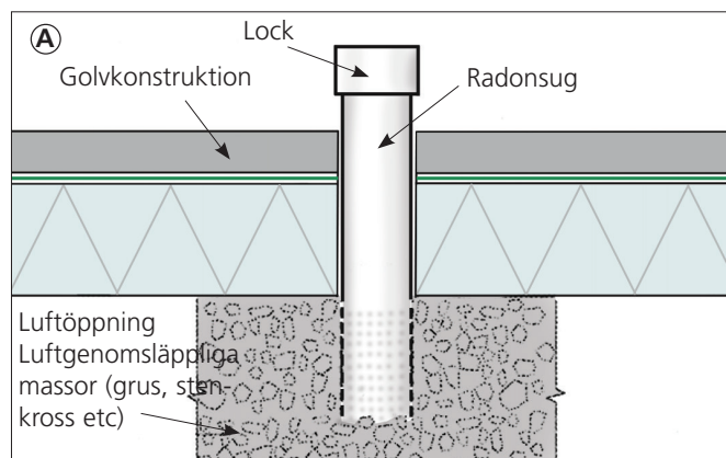
Principskiss, placering av radonsug
