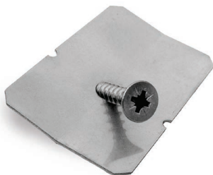
Fästskiva: (t=1 mm) 36 x 55 mm Skruv: 5 x 35 mm
